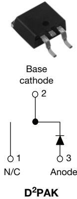
VS-MURB1520PbF
